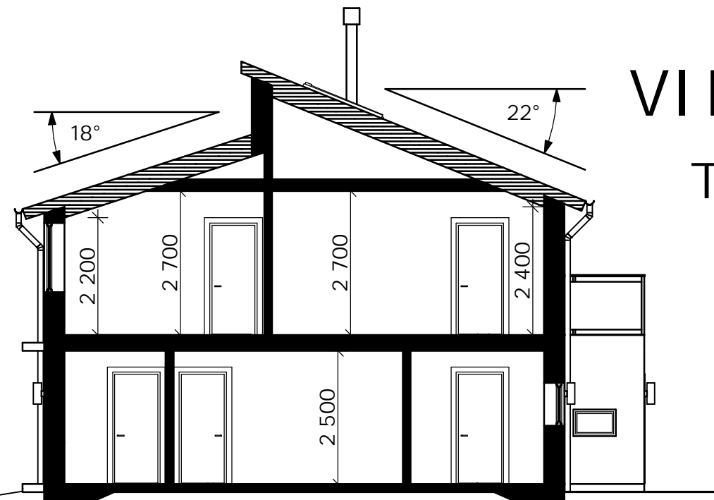
SEKTION B-B
