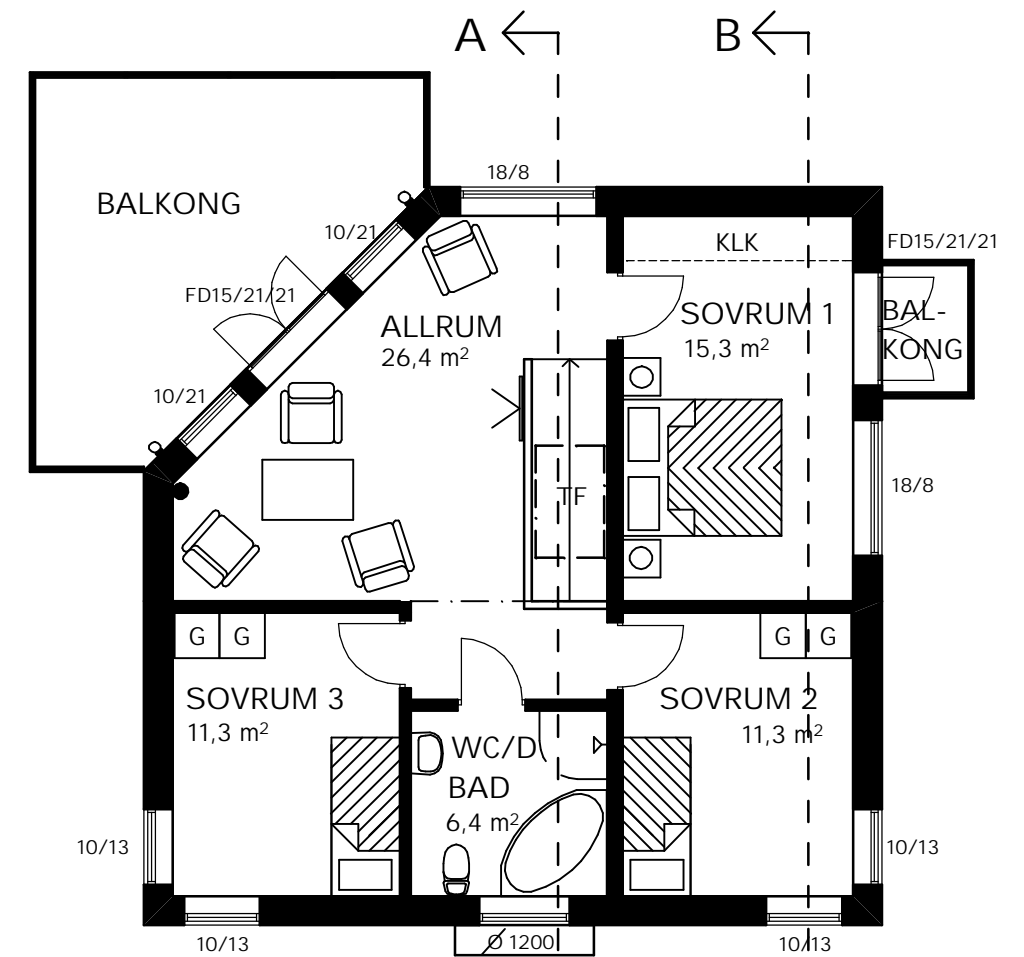
OVANPLAN Boyta: 74,7 m 2
