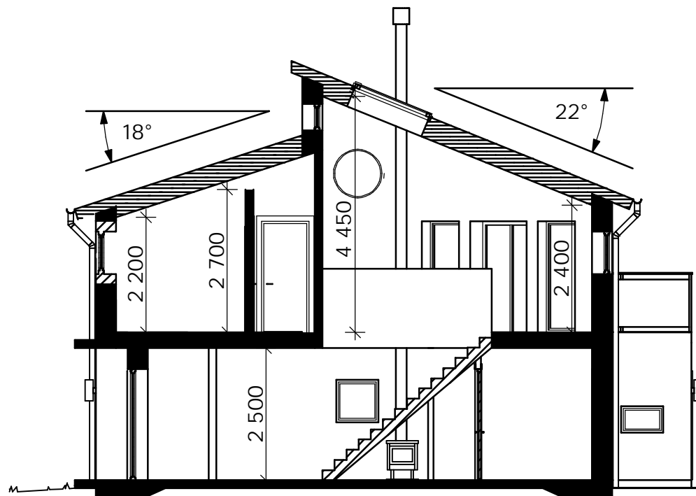
SEKTION A-A
